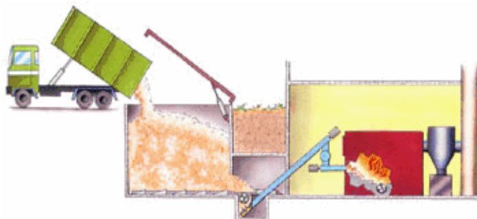
Prinsippskisse biokjel med brenslslager
